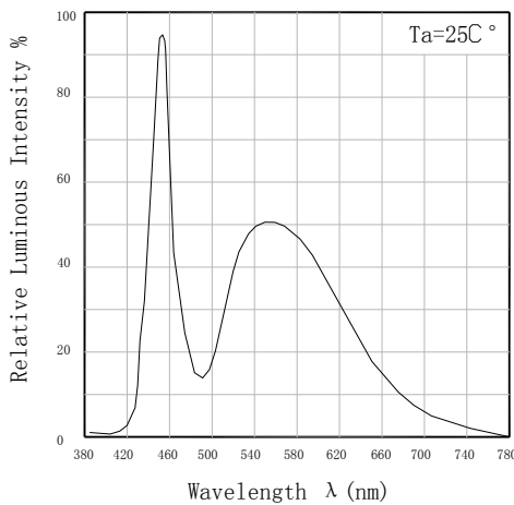
光谱特性图
