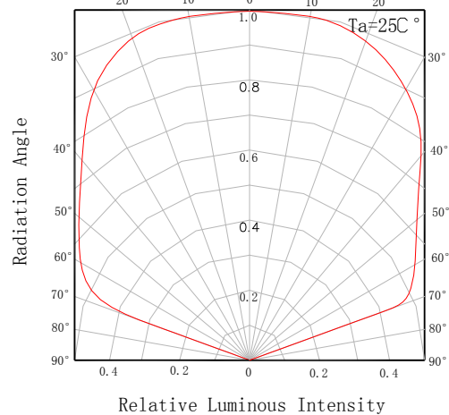
发光角度图
